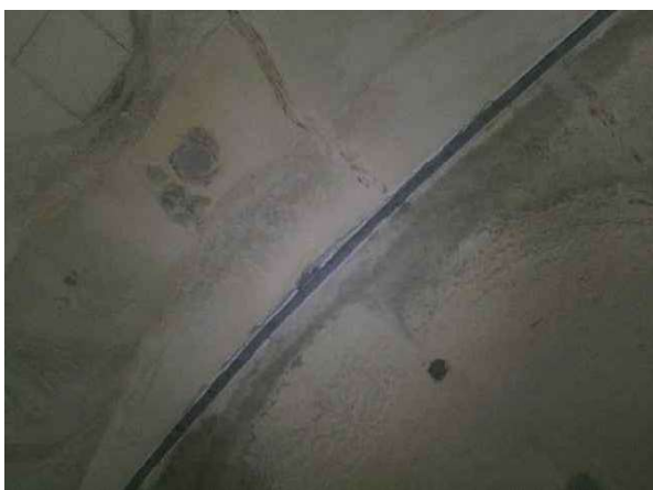
라이닝 S30 천단부 조인트부 들뜸-서울방향
