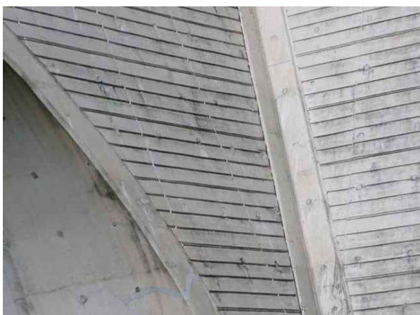
시점측 갭문 망상균열-문산방향
