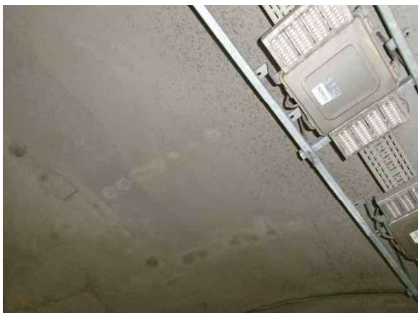
라이닝 S29 천단부 재균열(Cw=0.3mm이상)-서울방향
