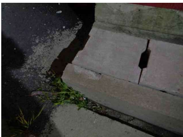
공동구 S12 파손-문산방향
