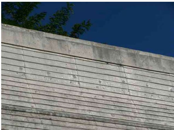
시점측 갭문 균열( C_w=0.3\text{mm} 미만)-서울방향
